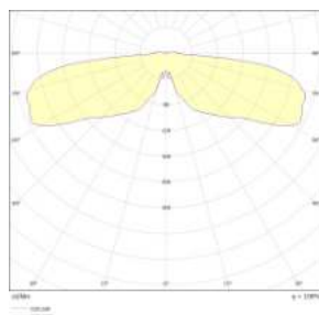
Lichtverdeling symmetrisch
